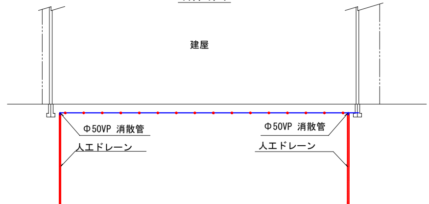
断面図
