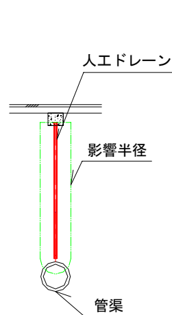
断面図
