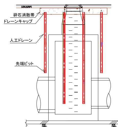
断面図
