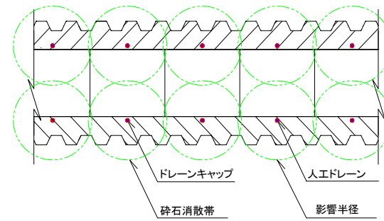
平面図
