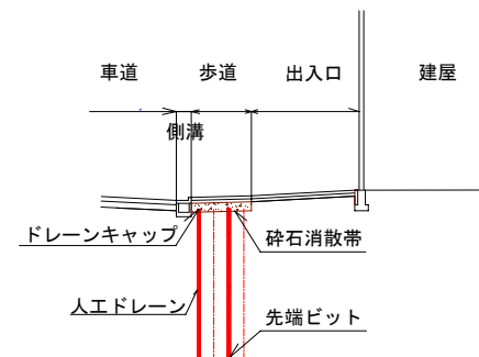
断面図 (A ~ A)
