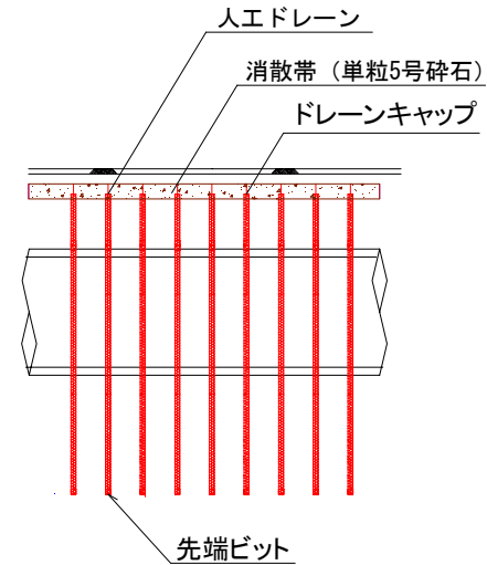
断面図
