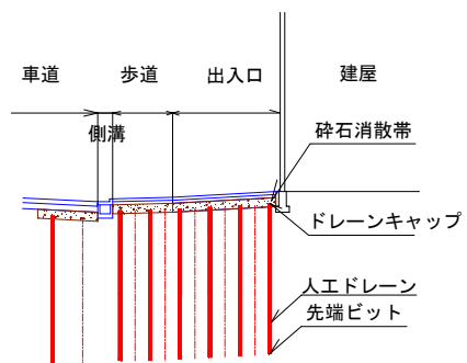
断面図 (A ~ A)
